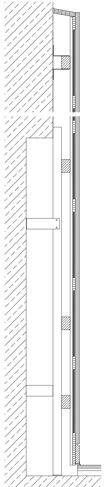
Weitspannträger
